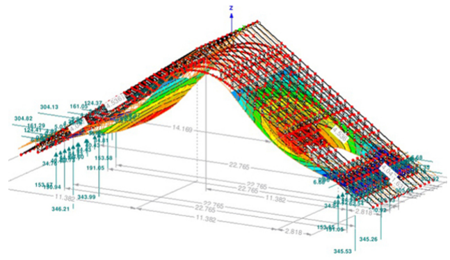
Modèle statique de la structure du toit
