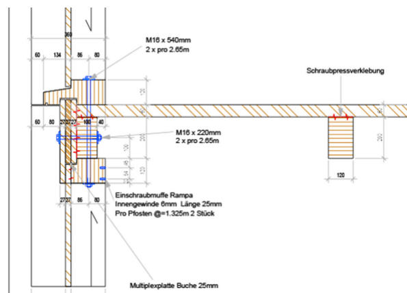
Détail de raccordement : mur extérieur-plafond d'étage
