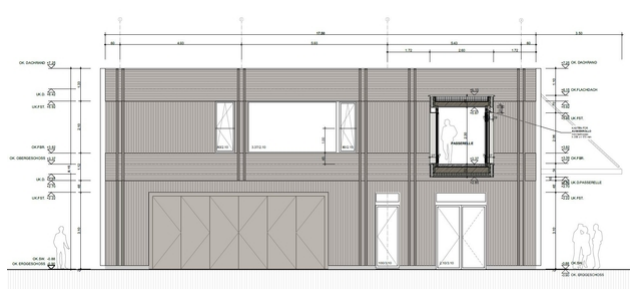
Westfassade
