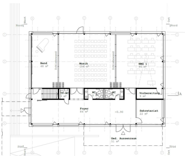
Grundriss Mehrzweckraum
